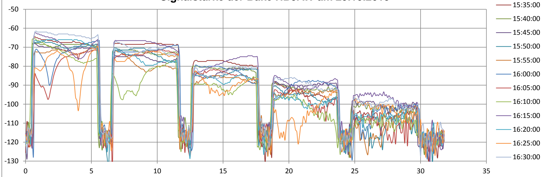
Signalstärke der Bake HB9AW am 29.10.2015
