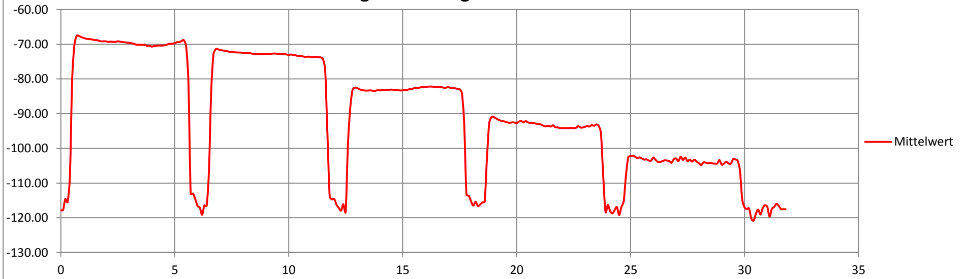
Gemittelte Signalleistung von HB9AW am 29.10.2015
